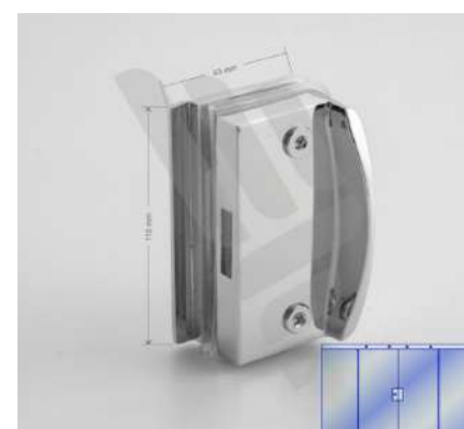
1511XJ - Contra fechadura 1510XJ para janela
