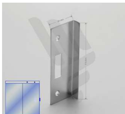
1511AX - Testeira fechadura para alvenaria 1510X
