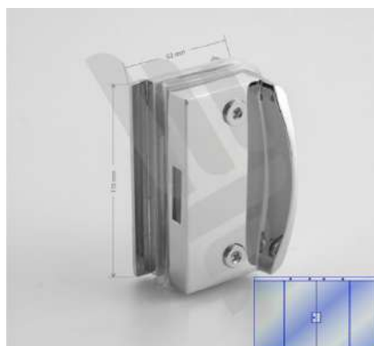
1511X - Contrafechadura para 1510X
