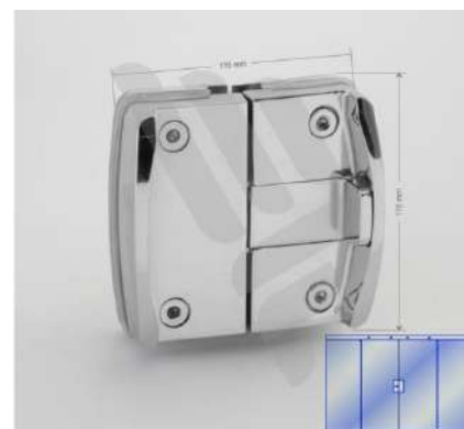
1570G - Fechadura central para janela sem miolo
