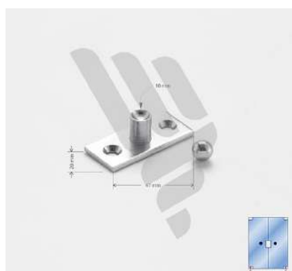
1014 - Pivô para dobradiça inferior
