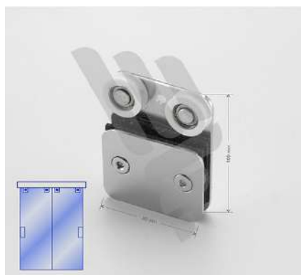
1126AC - Carrinho duplo 2 roldanas côncava
