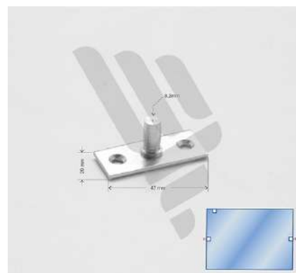
1009 - Pivô em aço para dobradiça superior
