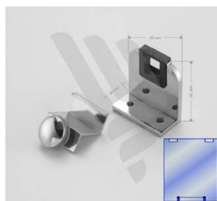
1587A - Conjunto acessório VA
